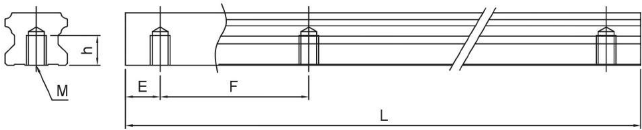
圖 2.2.4 下鎖式滑軌尺寸圖
